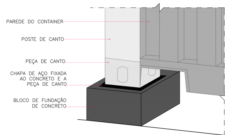
DETALHE DA FIXAÇÃO DO CONTAINER À FUNDAÇÃO
