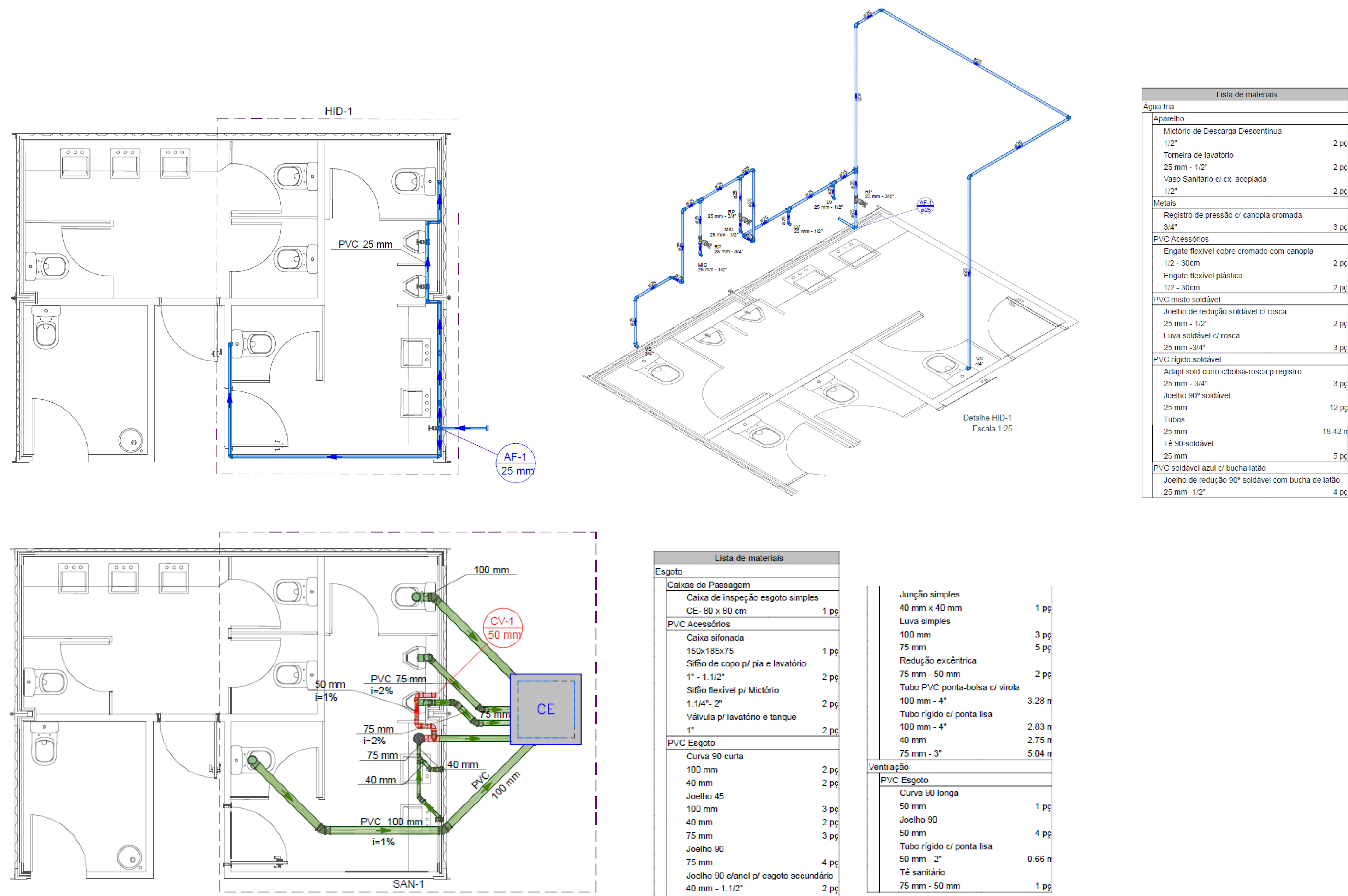
Figura 86, 87 e 88: Detalhamento 01 Fonte: Thais Ribeiro, (2022)
