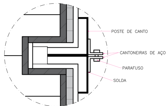
DETALHE 03
