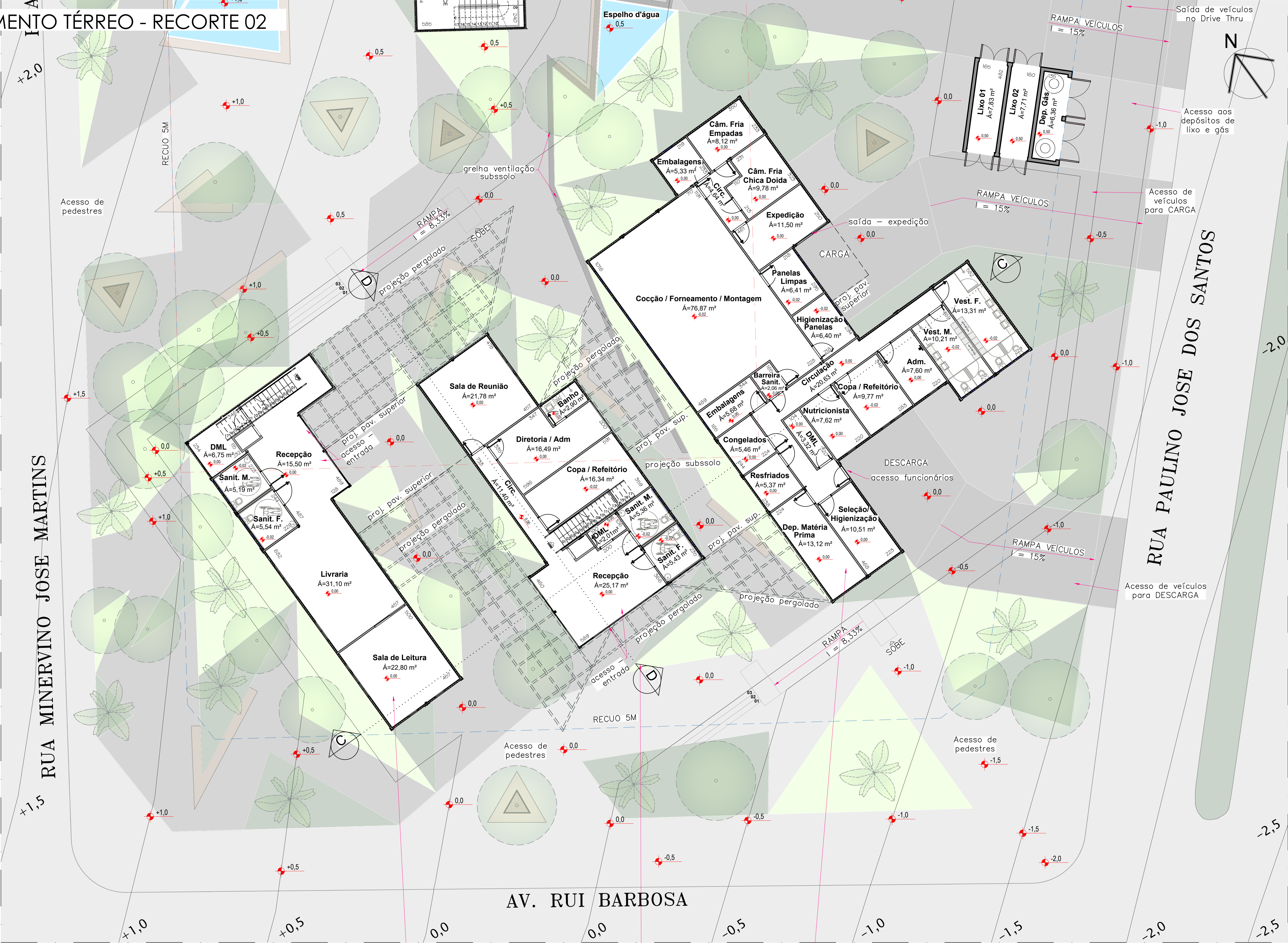
Figura 103: Planta CHAVE - Recorte 02 Fonte: Thais Ribeiro, (2022)
