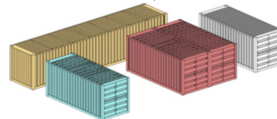
Figura 24: Planta térreo - disposição dos containers Fonte: Archdaily Edição: Thais Ribeiro, (2021)
