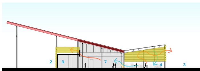
Figura 35: Esquema de ventilação
