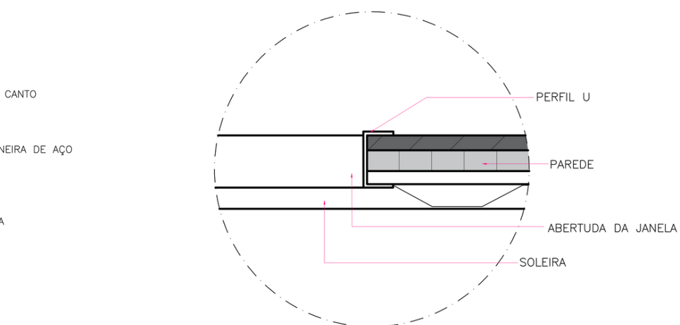
DETALHE 04
