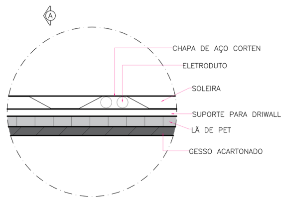
DETALHE 01
